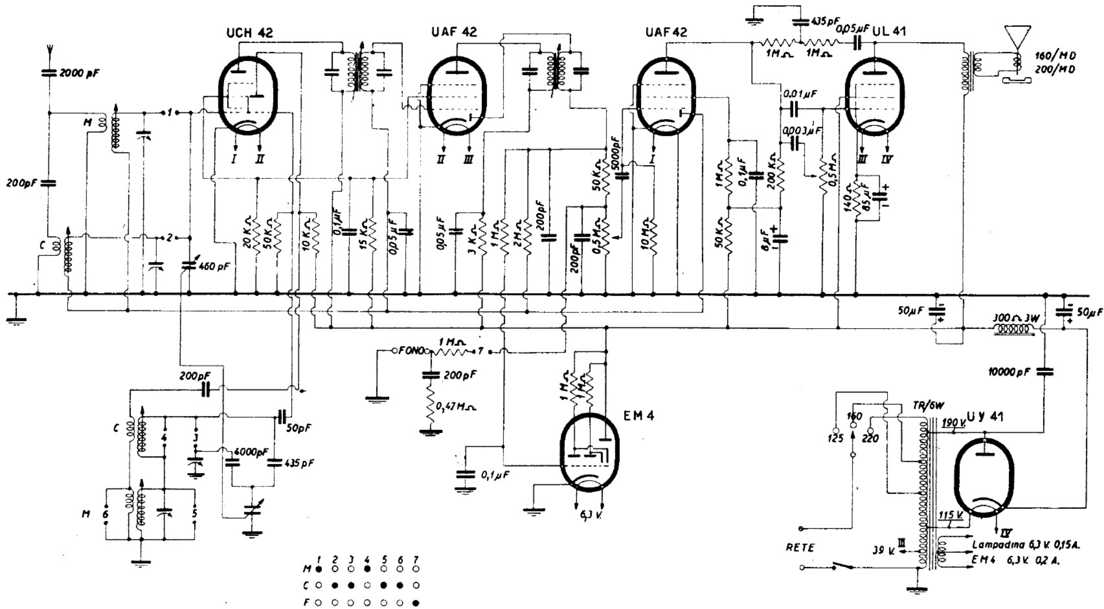
PEBA RADIO (Pertusati) - Mod. E 502/F. Caratteristiche uguali al mod. E 502, soprammobile fornito di riproduttore fonografico a tre velocità.
